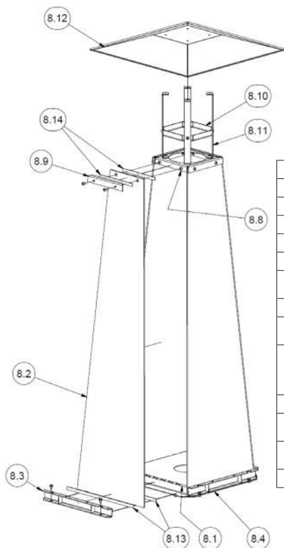
Slika 4. Shema postavljanja vrtne grijalice UMBRELLA/BS
