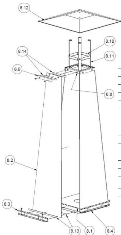
4. ábra Az UMBRELLA/BS kerti fűtőtest beépítési rajza
