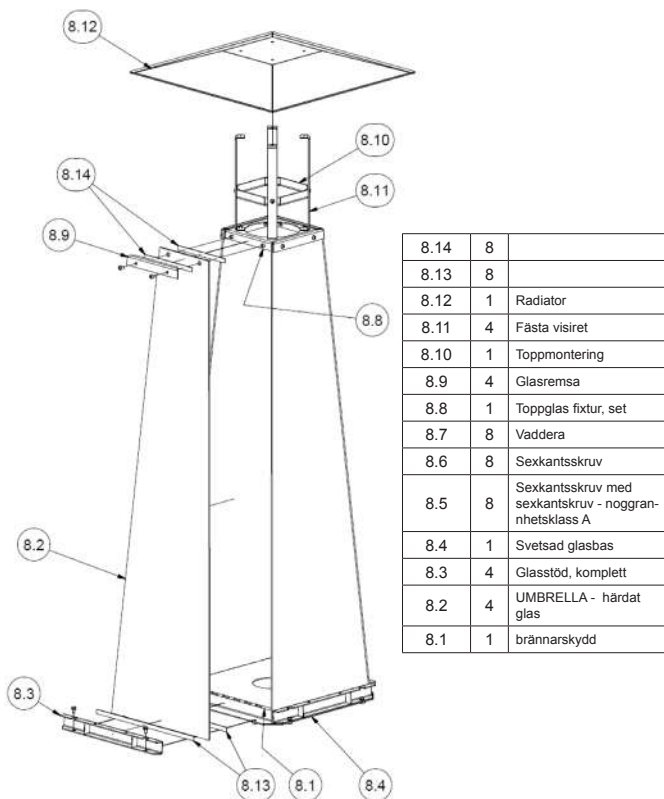
Fig. 4. Diagram över UMBRELLA / BS trädgårdsvärmare
