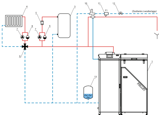
Schemat ogólny podłączenia kotła do instalacji c.o. i c.w.u w układzie zamkniętym zabezpieczony przed przegrzaniem zaworem termostatycznym SYR.
