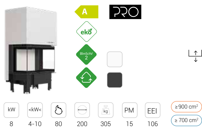
VN 480 787x494x329
