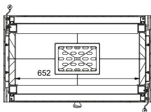
B-B (1 : 10)
