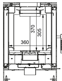
A-A (1 : 10)
