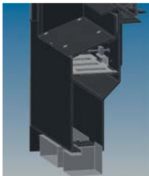
Rys.3 a) dolot powietrza pierwotnego b) kurtyna powietrzna
