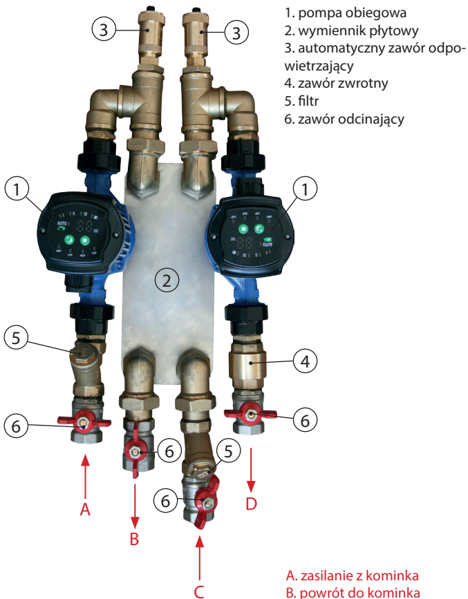
Rysunek 1. Schemat budowy zestawu mosiężnego wymiennikowo- płytowego.
