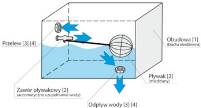
Rys. 2 Naczynie zbiorcze
